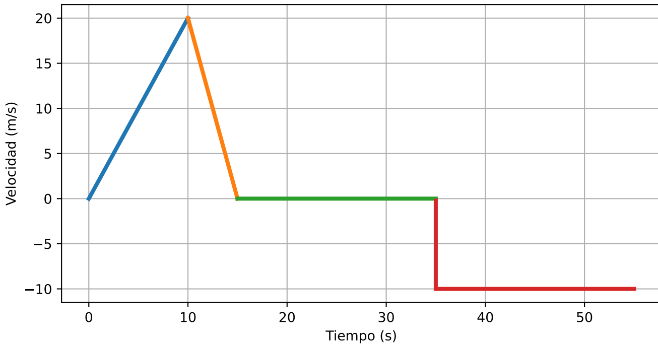
MRUA: Velocidad-tiempo
